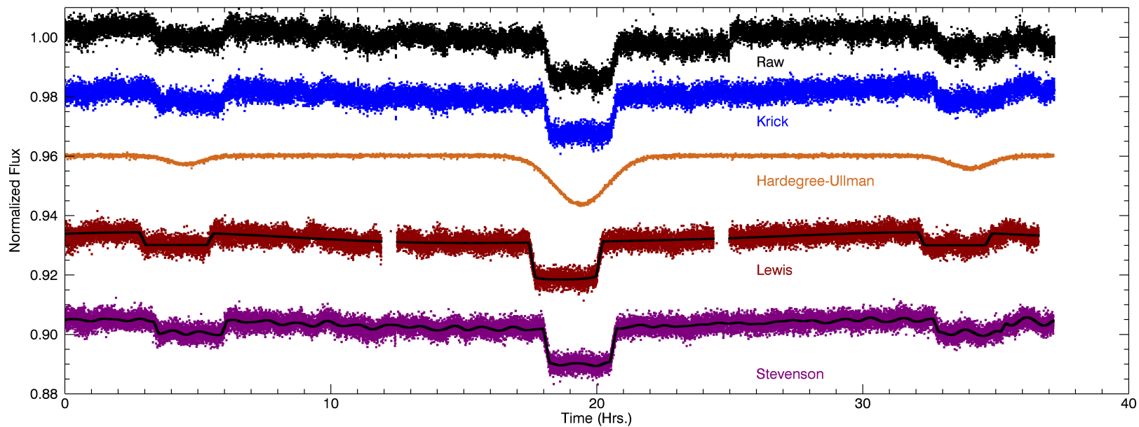
WASP-33b
