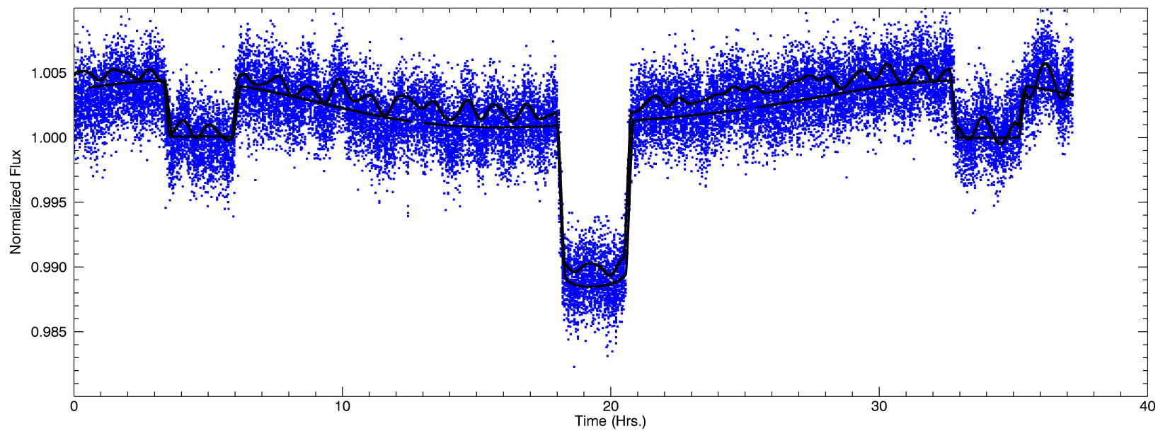
WASP-33b
