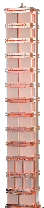
Cuoricino: \approx 1 CUORE tower
